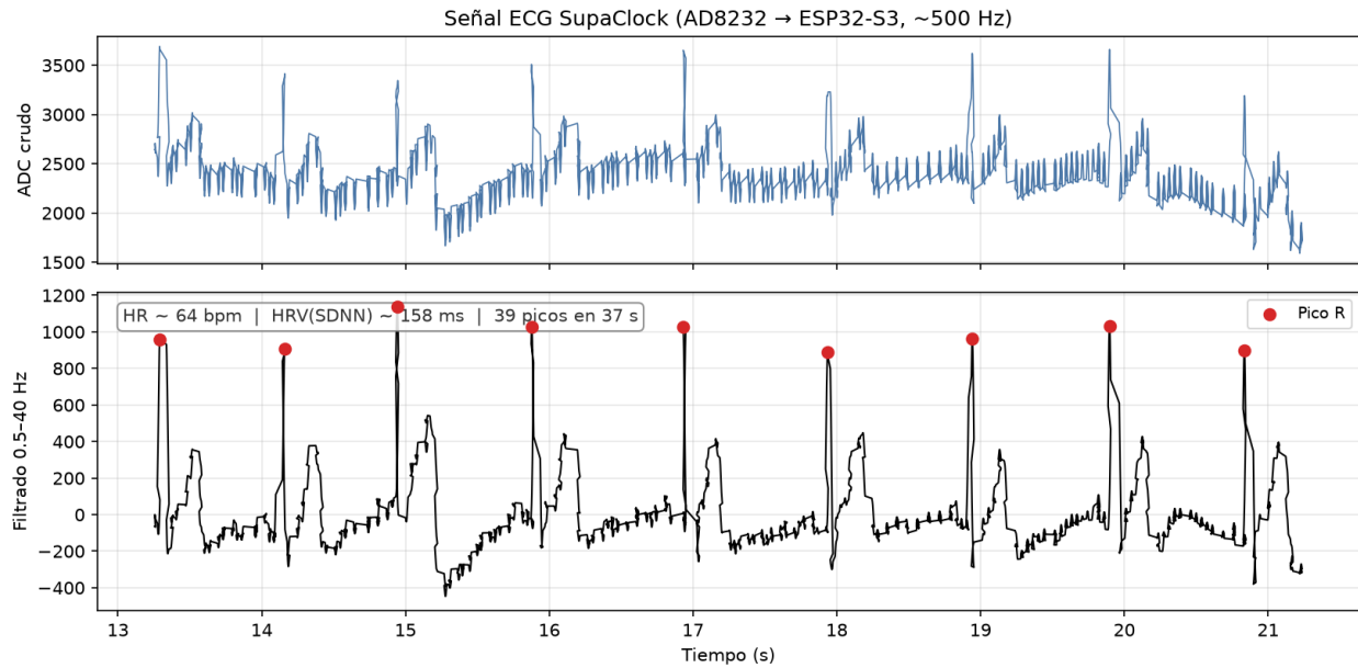
Figura 6: Señal ECG SupaClock (AD8232 \rightarrow ESP32-S3, \sim 500 Hz) con detección de picos R por el pipeline Pan-Tompkins app-side. El panel superior muestra la señal cruda del ADC, el inferior la señal filtrada 0,5–40 Hz con los 39 picos detectados en 37 s marcados en rojo. HR estimada \sim 64 bpm; HRV(SDNN) \sim 158 ms.
